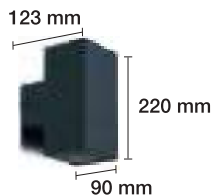
APLIQUE LED 6W PARED IP54 PF>0,9 DOBLE LUZ
